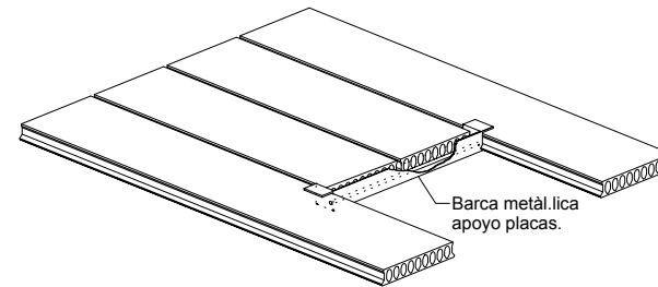
APOYO PLACA ALVEOLAR SOBRE BARCA METÁLICA
