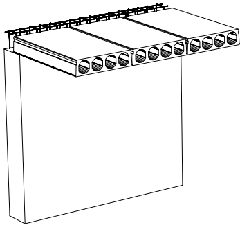
APOYO PLACA ALVEOLAR SOBRE MURO IN SITU
