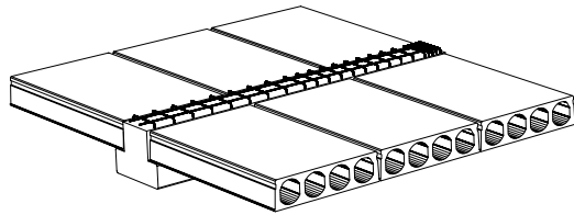
APOYO PLACA ALVEOLAR SOBRE JÁCENA TI
