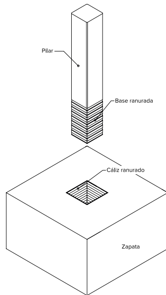
EMPOTRAMIENTO CON CÁLIZ RANURADO
