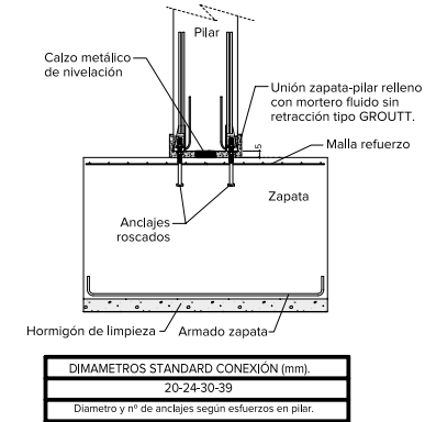
EMPOTRAMIENTO CON ANCLAJES ROSCADOS
