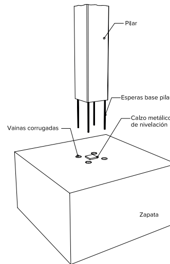
EMPOTRAMIENTO CON VAINAS CORRUGADAS
