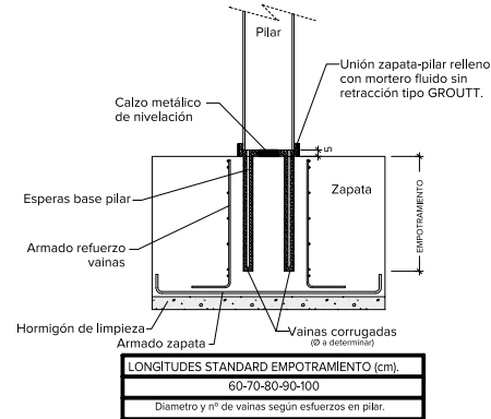
EMPOTRAMIENTO CON VAINAS CORRUGADAS
