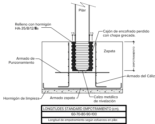
EMPOTRAMIENTO CON CÁLIZ RANURADO
